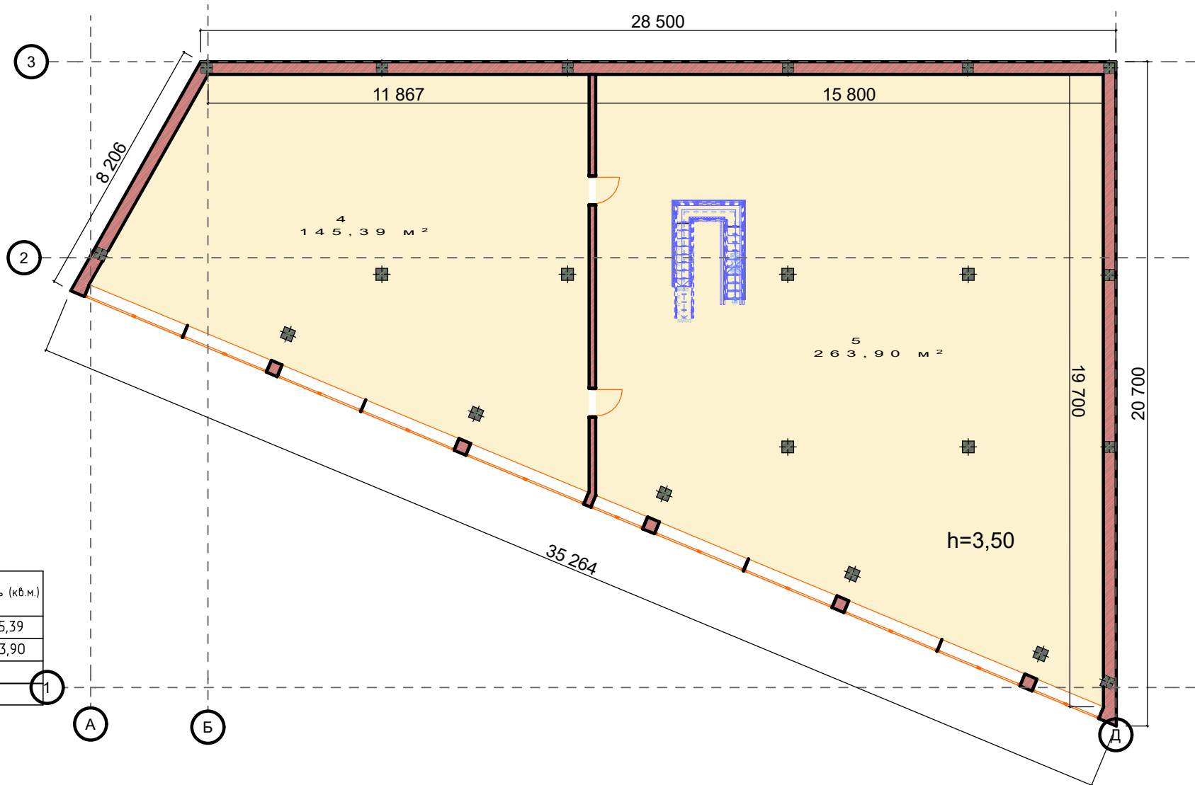
Экспликация 2 этажа
