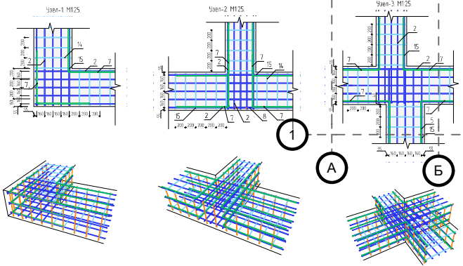
Схема армирования
